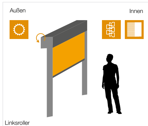
Basisausführung bei zipSCREEN.2, zipSCREEN F50, PURO 2.XR-zip mit Führungsschiene 33x61 mm und rollSCREEN.2
